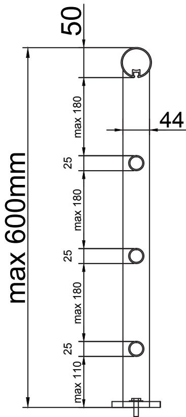
VOETPLAAT 80X100X10
